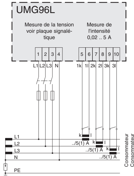
Fig.: Exemple de raccordement 7 Mesure dans le réseau IT par le biais de trois transformateurs d'intensité.
