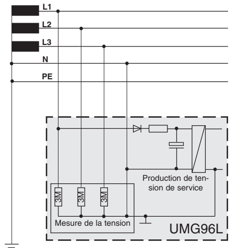
Fig. Acquisition de la tension de service à partir de la tension de mesure.
